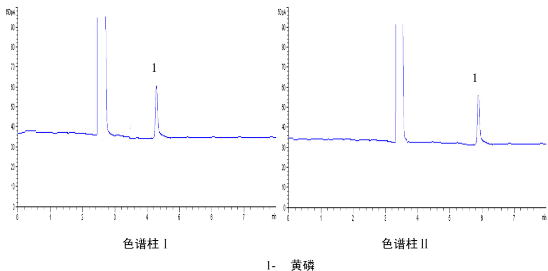
图 1 黄磷色谱图（NPD 检测器）
